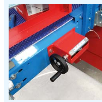
4 Dispositivo de ajuste para bandejas con pie.
