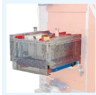
3 Distribuidor electroneumático con 3 movimientos para bandejas termoformadas en PE - PET.
