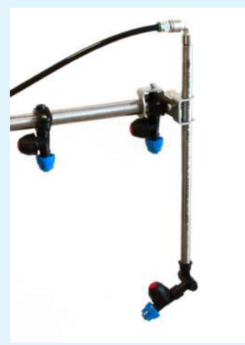
Boquilla de articulación independiente , con brazo de acero inoxidable regulable en altura , con válvula para el riego de los bordes.
