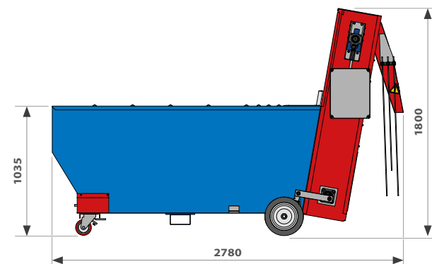
TR1800 en la función de “pulmón” para el sustrato, insertada entre CARBB y RN12, completa con cinta transportadora mod. NTV on patas especiales y lados laterales.
